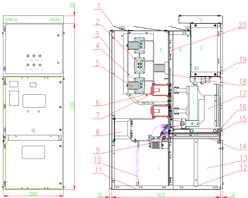
图 1 KYH1-24 馈线开关柜基本结构剖面图
