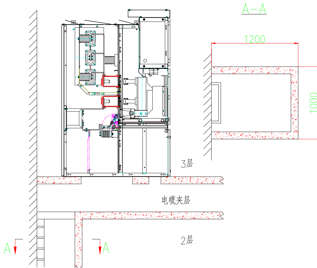
图 4 楼上安装示意图
